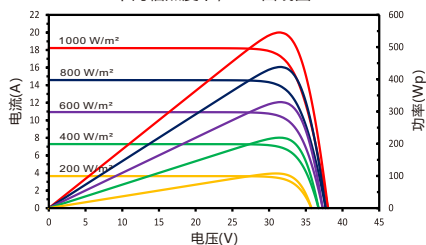
RSM110-8-545M 不同辐照度下, I-V 曲线图
